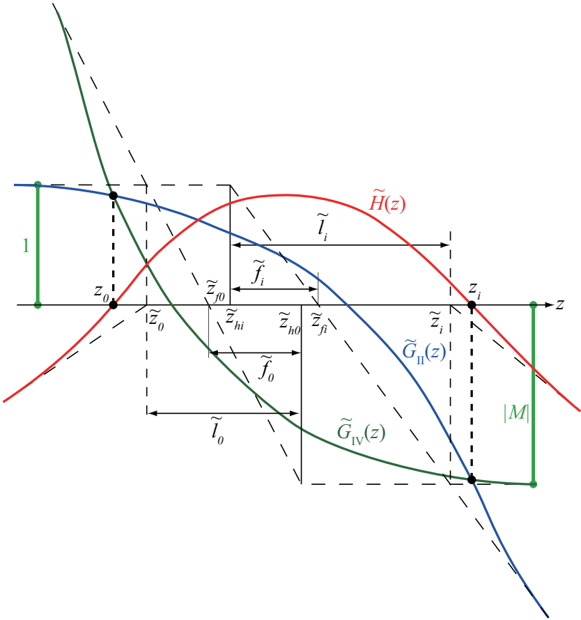
図 1 物と像の両方が漸近結像の時
