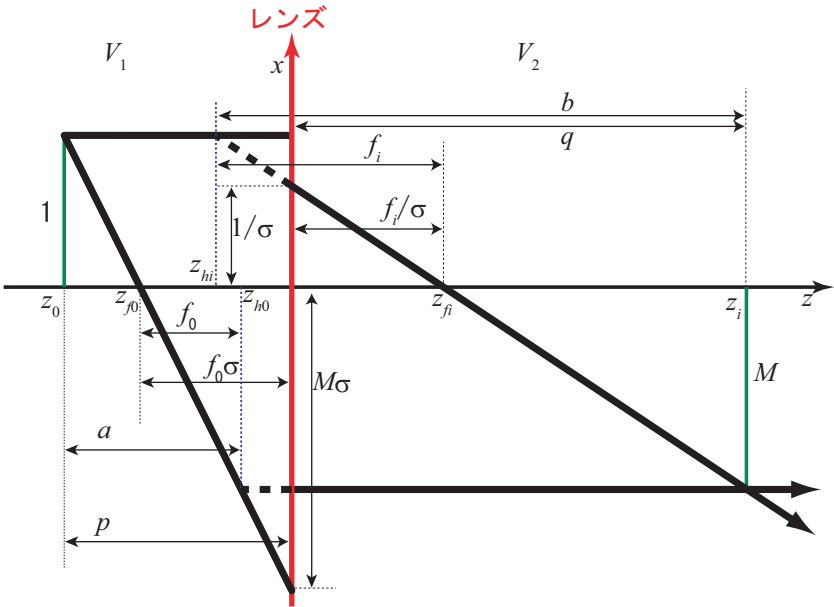
図3 バイポテンシャルレンズの薄肉近似光線図。 \sigma = 3/2 , |M| = 4/3 , f_i/\sigma = f_0\sigma = 1 の時の作図。
