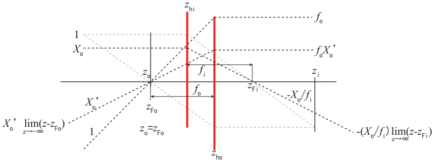
図5 式 (16.15)～式 (16.17) の文字の説明のための薄肉近似光線図。(参考: 図 4.26)
