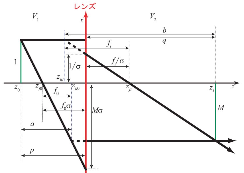
図3 バイポテンシャルレンズの薄肉近似光線図。 \sigma = 3/2 , |M| = 4/3 , f_i/\sigma = f_0\sigma = 1 の時の作図。
