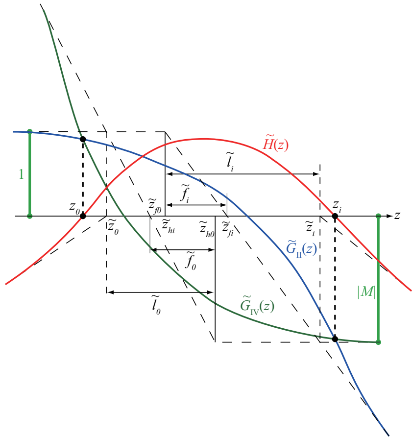
図1 物と像の両方が漸近結像の時
