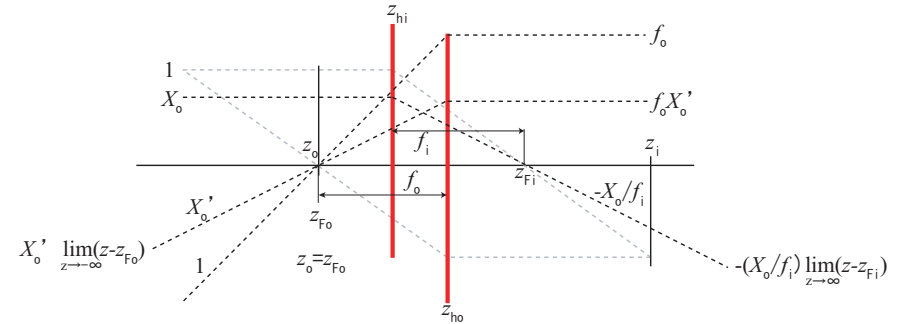
図 5 式 (16.15)~ 式 (16.17) の文字の説明のための薄肉近似光線図。(参考: 図 4.26)
