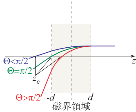
図2 均一磁界モデルでの軌道 ( |M| \gg 1 )
