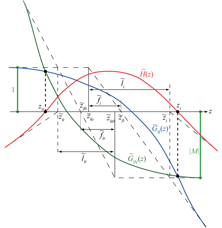
図 1 物と像の両方が漸近結像の時
