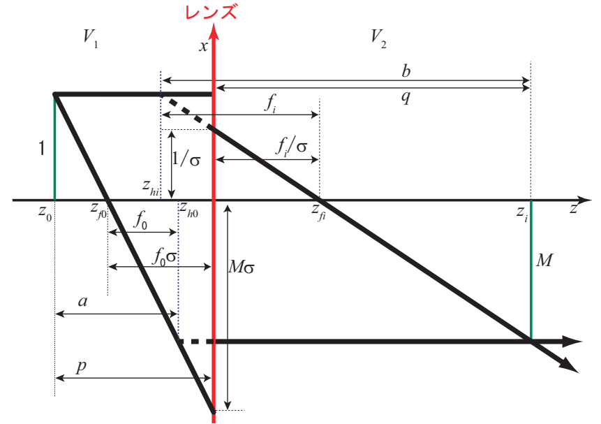
図3 パイポテンシャルレンズの薄肉近似光線図。 \sigma = 3/2 , |M| = 4/3 , f_i/\sigma = f_0\sigma = 1 の時の作図。
